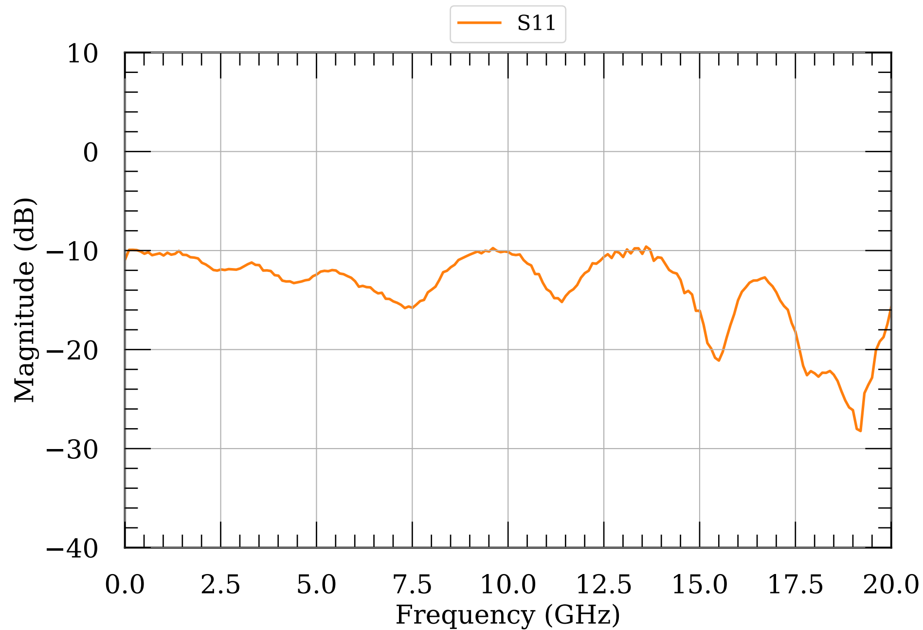
LNA S-params module097
